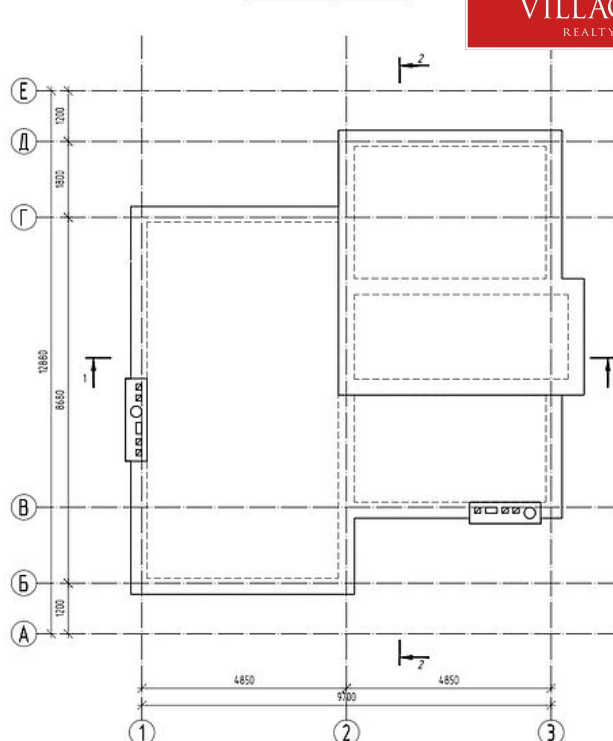
План кровли
