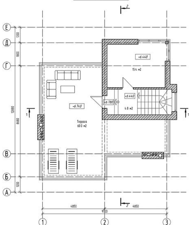
План 3 этажа
