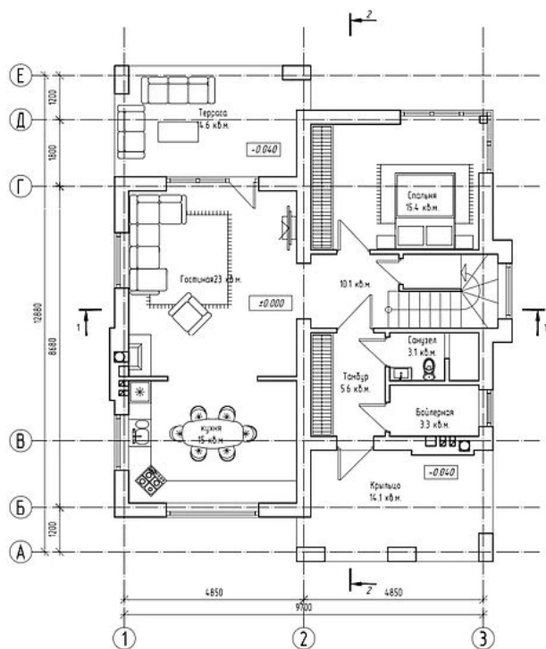
План 1 этажа
