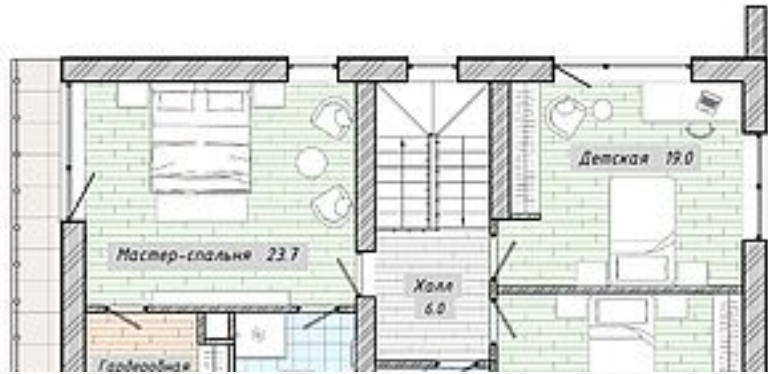
План 2 этажа
