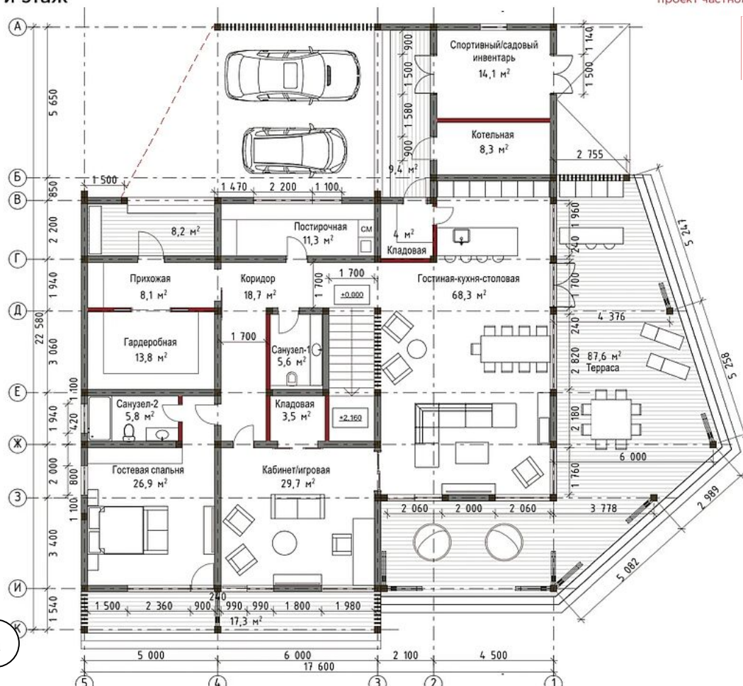
План дома / 1-й этаж
