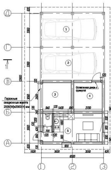
ПЛАН НАВЕСА С ХОЗБЛОКОМ
