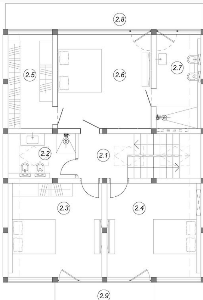
План второго этажа
