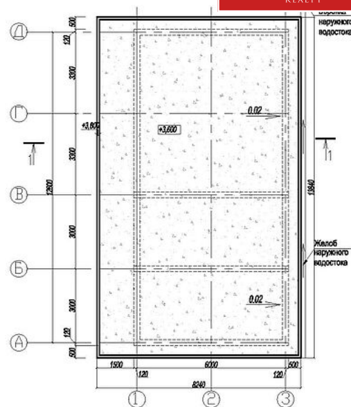
ПЛАН КРОВ
