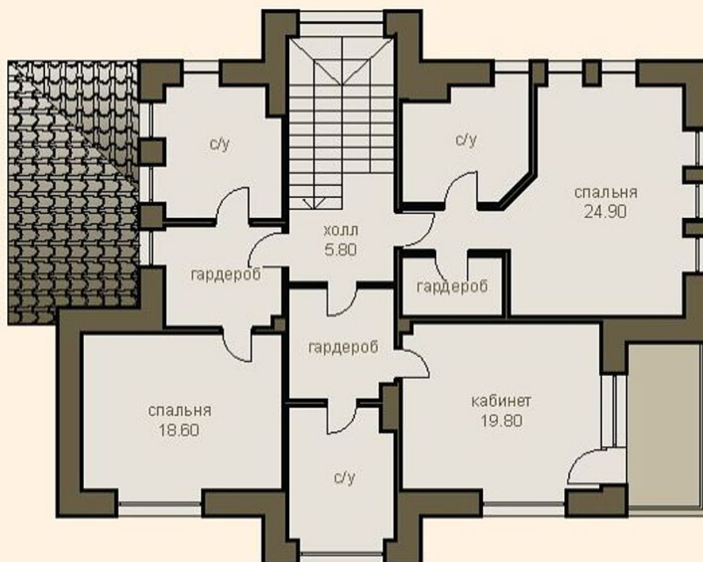
План-схема
