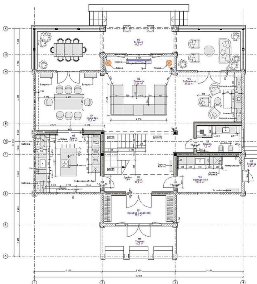
План 1 этажа
