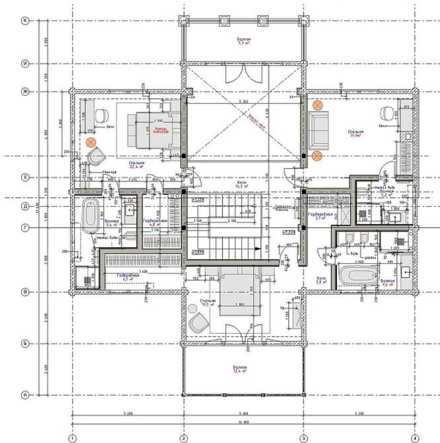
План 2 этажа
